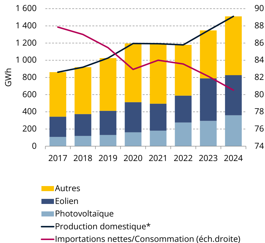
Production et consommation d'électricité au Luxembourg
