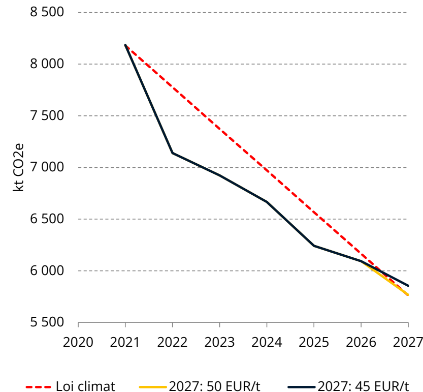
Emissions de GES pour différents niveaux de taxe CO 2
